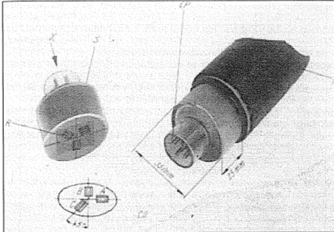
Fig. 10.—A la izquierda, «doorstopper» en el que se aprecia la roseta de extensómetros. A la derecha, «doorstopper» pegado a un testigo. R: roseta de bandas extensométricas; S: Lámina de plástico; D: Testigo CG: Configuración de los extensómetros en el fondo del taladro, visto en la dirección del eje x. (Leeman, 1971)
