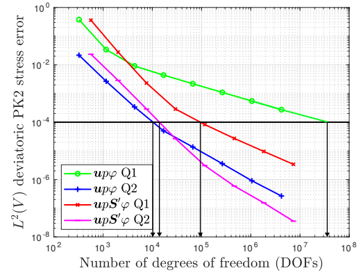
(D) Deviatoric PK2 mechanical stress error upon DOFs
