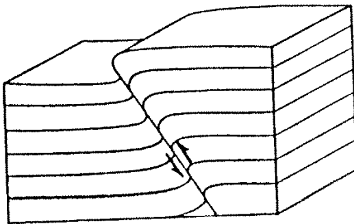
FALLA INVERSA
