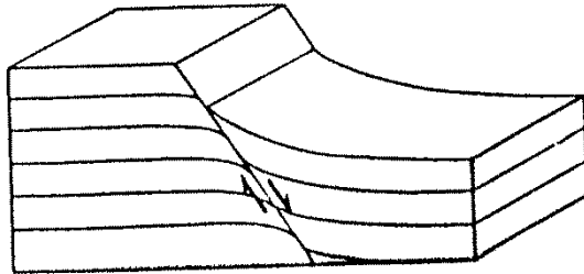
FALLA NORMAL
